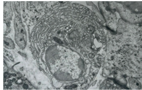
Рисунок 2 – Ядрышки сегрегированы
