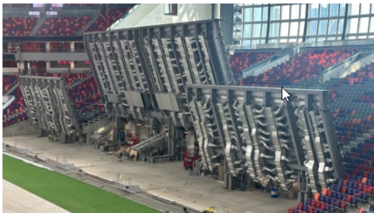
Рисунок 3 – Трансформируемые архитектурно-конструктивные решения
