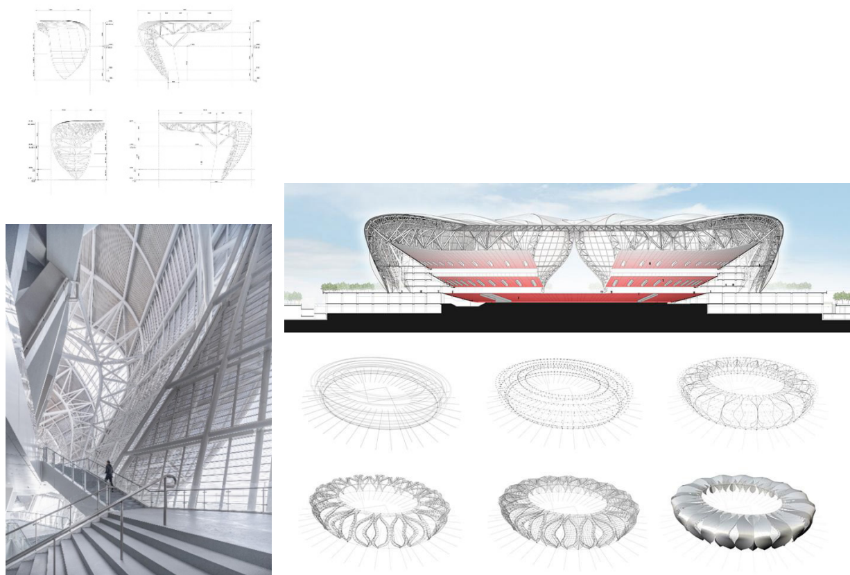
Рисунок 1 – Ограждающая конструкция стадиона
