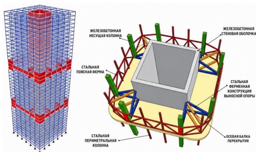
Рисунок 4 – Принципиальное конструктивное решение аутригерной системы высотного здания
