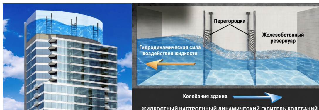
Рисунок 3 – Конструктивное решение TLD
