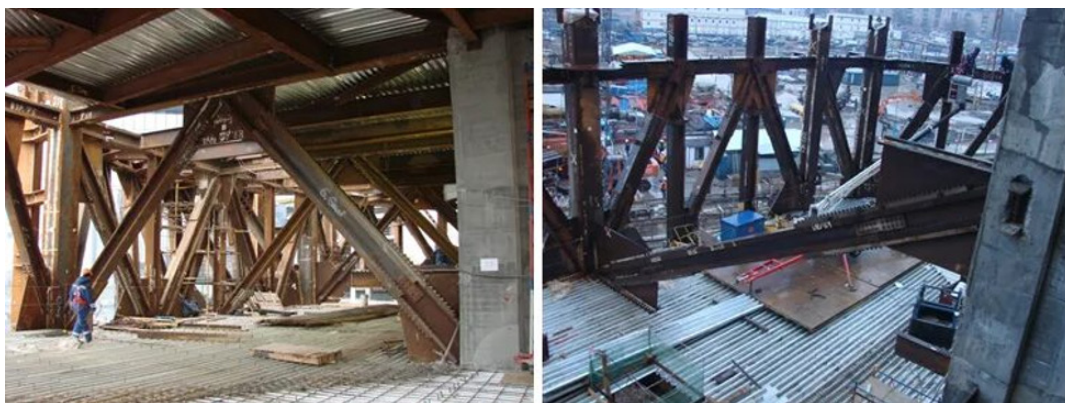
Рисунок 5 – Конструктивные элементы аутриггерной системы (балки, стойки, раскосы-демпферы) [12]
