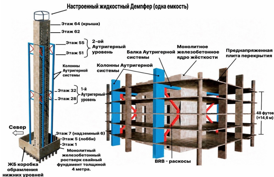
Рисунок 2 – Конструктивное решение Южной башни One Rincon Hill (на рисунке не отображены натянутые внутри ядра стальные тросы)
