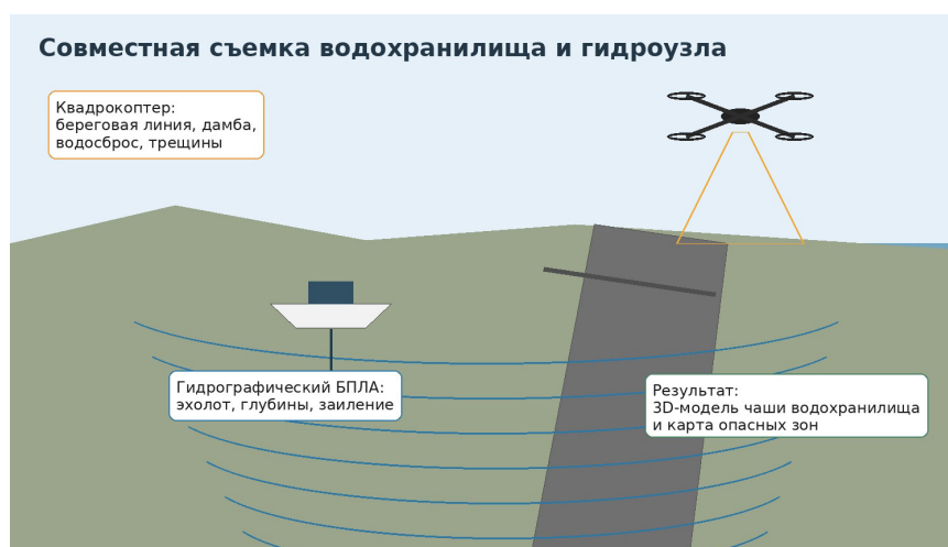
Рисунок 7 – Иллюстративная схема совместной съемки водохранилища: квадрокоптер контролирует надводные элементы, гидрографический БПЛА выполняет промер глубин
