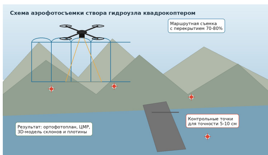
Рисунок 4 – Иллюстративная схема маршрутной аэрофотосъемки створа гидроузла квадрокоптером
