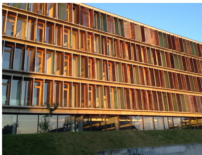
Рисунок 1 – Адаптивная фасадная оболочка с наружными солнцезащитными ламелями как средство регулирования инсоляции, бликов и визуального комфорта
