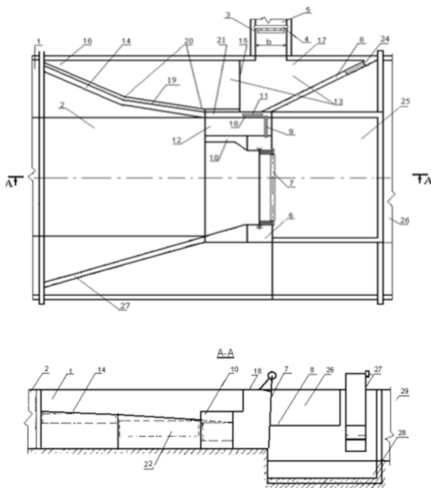
Рисунок 3 – Расчетная схема водозаборного гидроузла для деривационных ГЭС с ломаным в плане наносозащитным порогом
