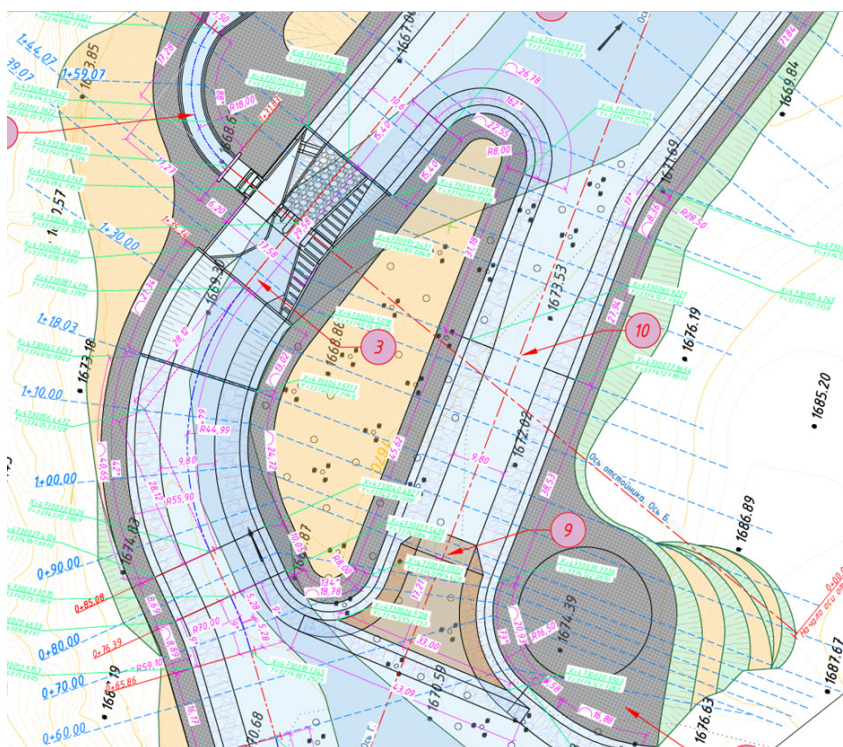
Рисунок 1 – Схема размещения головного водозаборного гидроузла усовершенствованной тянь-шаньской компоновки на участке р. Шамси
