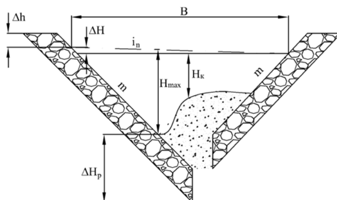
Рисунок 2 – Расчётная схема поперечного сечения криволинейного русла
