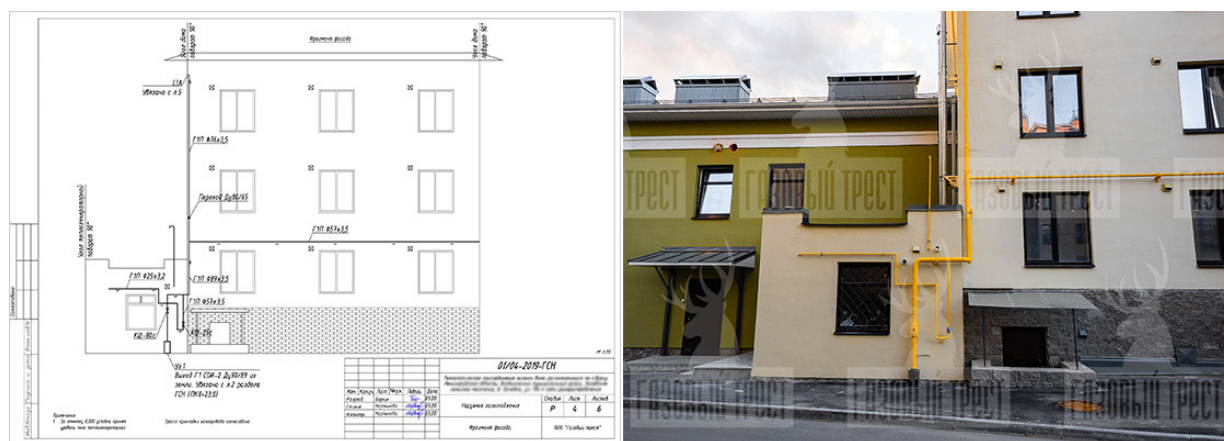
Рисунок 3 – Разводка внутридомовых газопроводов по фасаду здания
