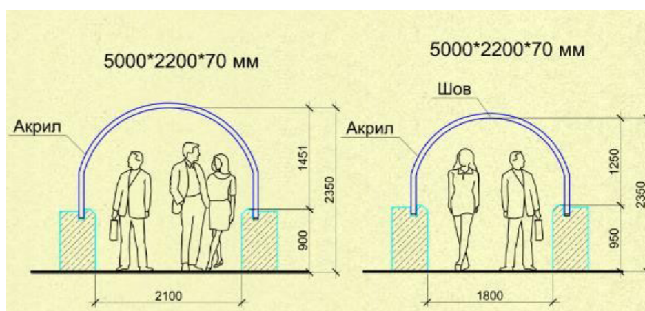
Рисунок 6 – Пример подводного тоннеля в экспозиции океанариума. Тоннель изготовлен из акриловых панелей цилиндрической формы с углом обзора \sim 180^\circ [12]
