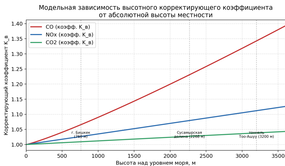
Рисунок 2 – Модельная зависимость высотного корректирующего коэффициента K в от абсолютной высоты местности для CO, NO x и CO 2
