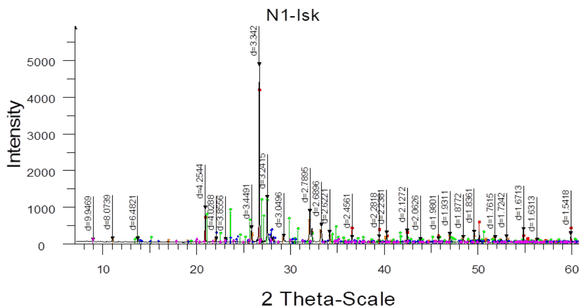
Рисунок 2 – Дифрактограмма концентрата фосфоритов месторождения Чилисай
