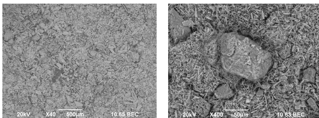
Рисунок 3 – Вид образовавшихся кристаллов фосфогипса при разном увеличении
