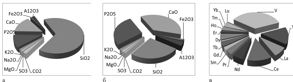
Рисунок 1 – Химический состав образцов исходной руды (а) и концентратов месторождения Чилисай (б, в)
