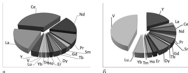
Рисунок 5 – Распределение редкоземельных элементов и ванадия, оставшихся в кеке (а) и перешедших в раствор (б)
