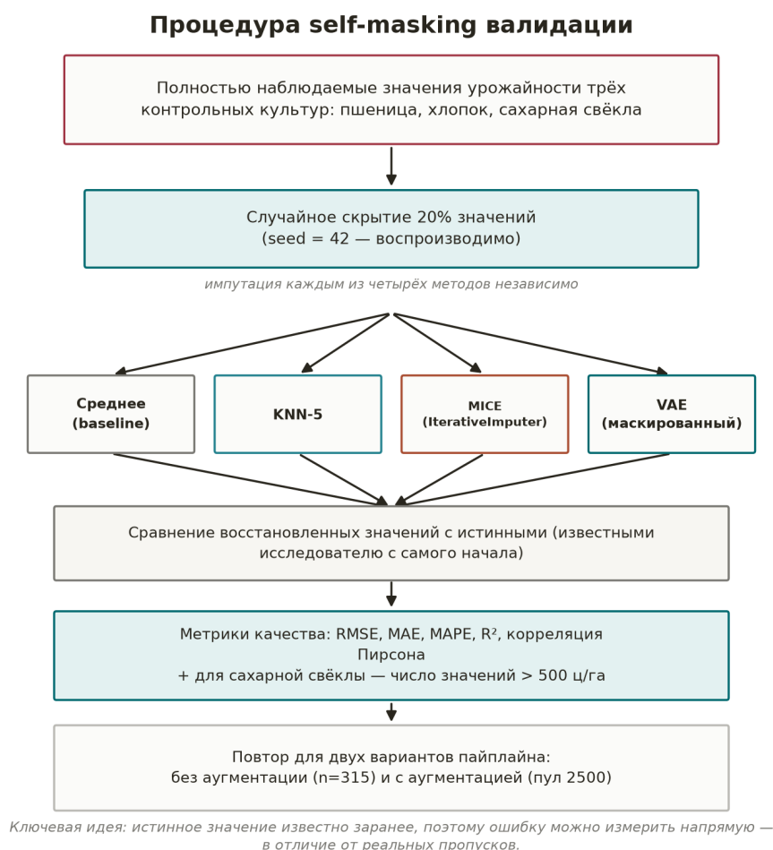
Рисунок 3 – Схема процедуры self-masking валидации: искусственное скрывание 20 % реально наблюдаемых значений, независимая импутация четырьмя методами, сравнение с истинными значениями и расчёт метрик качества
