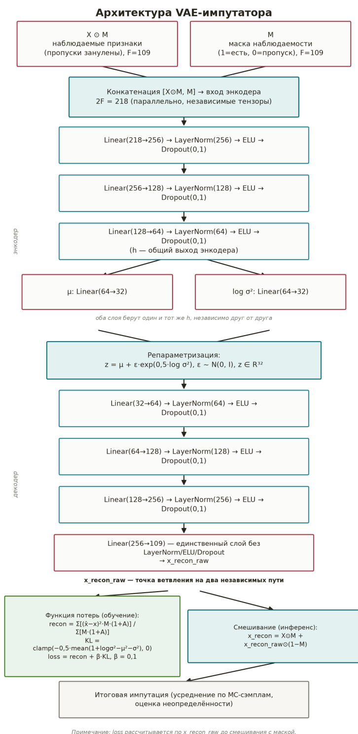
Рисунок 1 – Архитектура маскированного вариационного автоэнкодера: вход X \odot M и маска M , энкодер 2F \rightarrow 256 \rightarrow 128 \rightarrow 64 , латентное пространство (\mu, \log \sigma^2) размерности 32, декодер 64 \rightarrow 128 \rightarrow 256 \rightarrow F . Для используемой панели F = 109 , то есть 2F = 218
