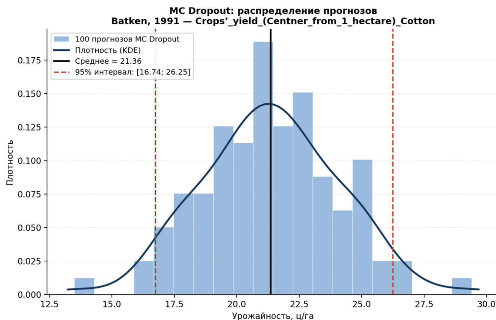
Рисунок 3 – Гистограмма 100 прогнозов MC Dropout для реально пропущенного значения (урожайность хлопка, Баткен, 1991 год; вариант с аугментацией): среднее – 21,36 ц/га, 95%-й интервал – (16,74; 26,25)
