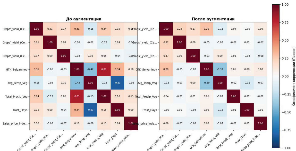
Рисунок 1 – Корреллограммы восьми ключевых признаков до и после аугментации (данный прогон): среднее абсолютное отклонение корреляций – 0,094
