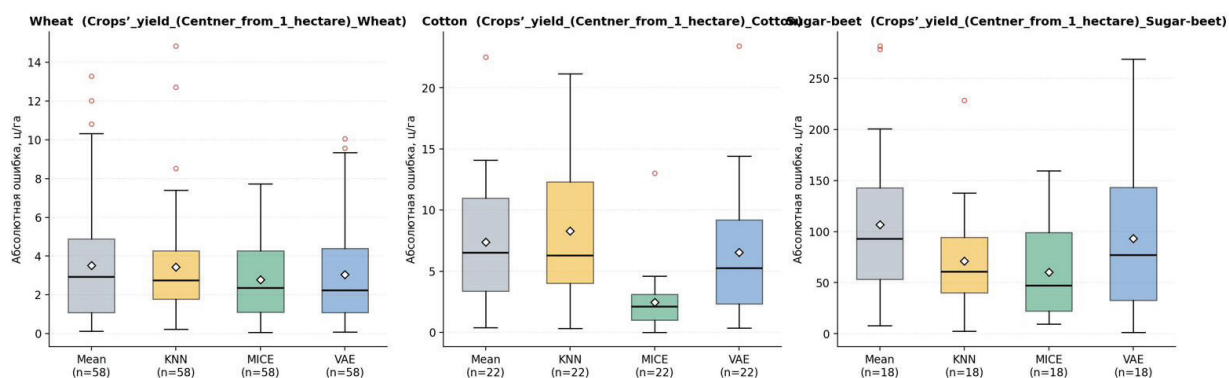
Рисунок 4 – Box-plot абсолютных ошибок self-masking восстановления по четырём методам (Mean, KNN, MICE, VAE) для трёх контрольных культур (вариант с аугментацией)
