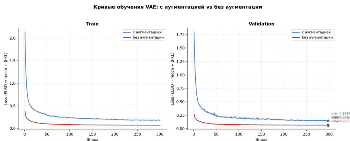
Рисунок 2 – Кривые обучения (ELBO: train/val) без аугментации и с аугментацией. Без аугментации loss выходит на существенно более низкий уровень (val \approx 0,062) по сравнению с аугментированным вариантом (val \approx 0,145)
