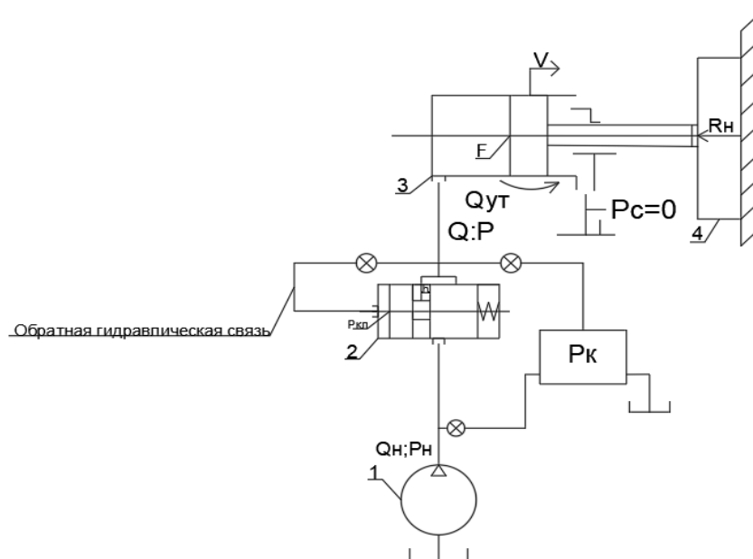
Рисунок 1 – Схема автоматического управления регулирования скорости:
