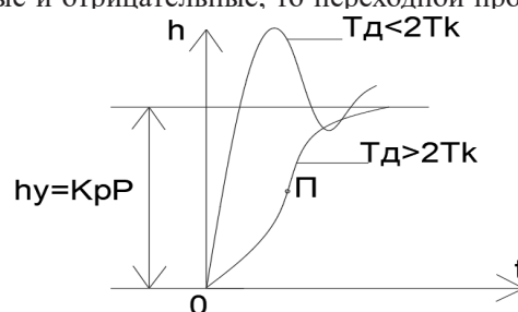
Рисунок 4 – Переходной процесс регулятора расхода
