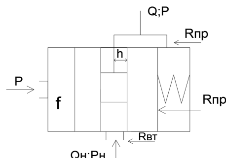
Рисунок 3 – Схема регулятора расхода
