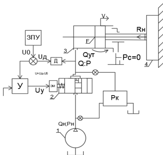
Рисунок 2 – Автоматическая система управления гидравлического пресса:
