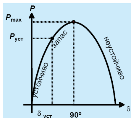
Рисунок 3 – Угловая характеристика мощности линии электропередачи
