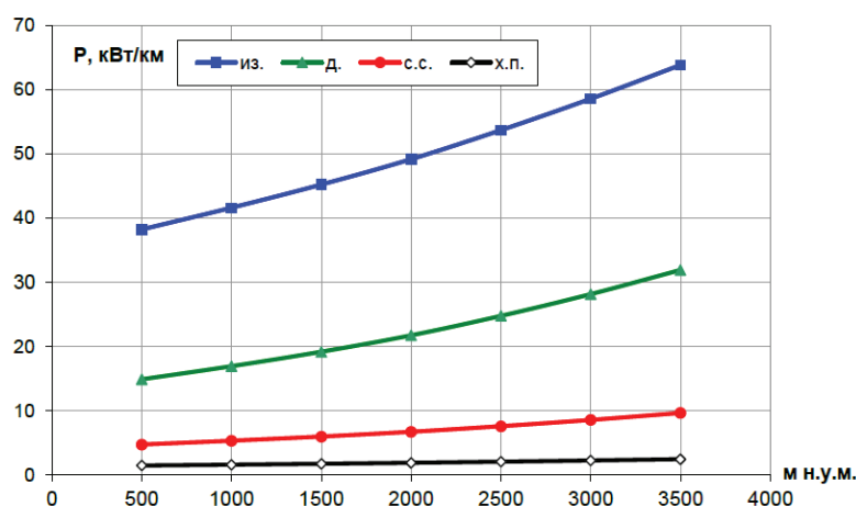
Рисунок 5 – Удельные потери мощности на корону для воздушной линии электропередачи напряжением 500 кВ, провод АС-3 × 300
