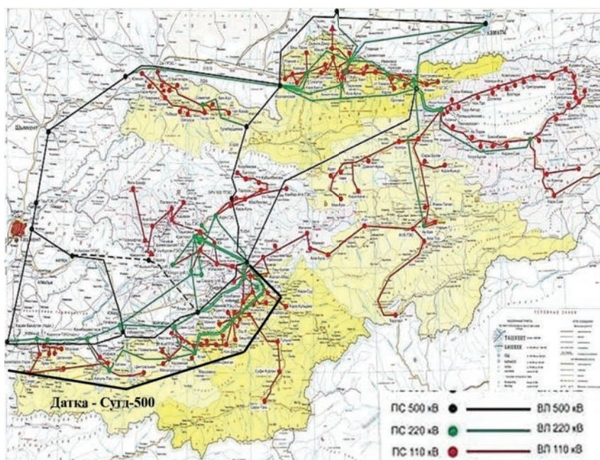
Рисунок 1 – Схема основных сетей 110–500 кВ энергосистемы Кыргызстана
