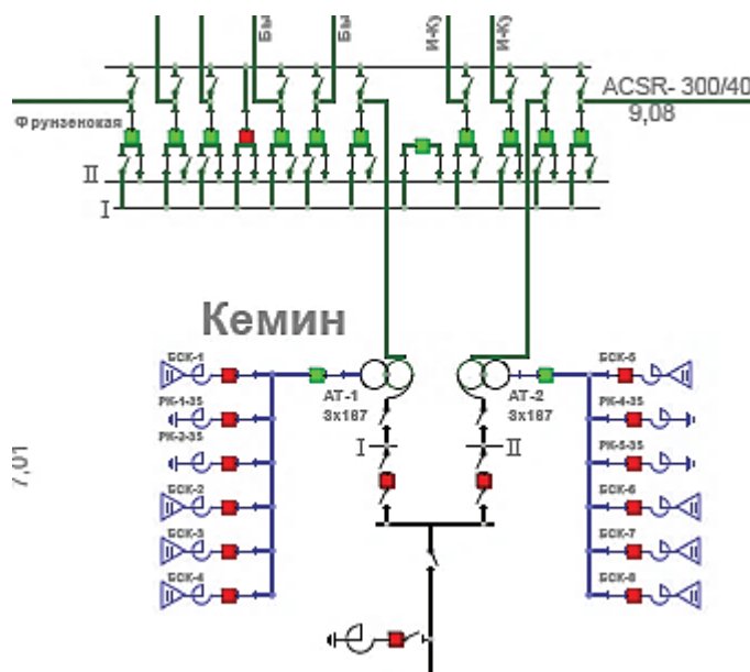
Рисунок 4 – Схема подключения БСК на подстанции «Кемин»
