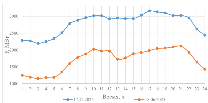
Рисунок 2 – Суточные графики нагрузок летнего и зимнего режимов энергосистемы Кыргызстана за 2025 г.
