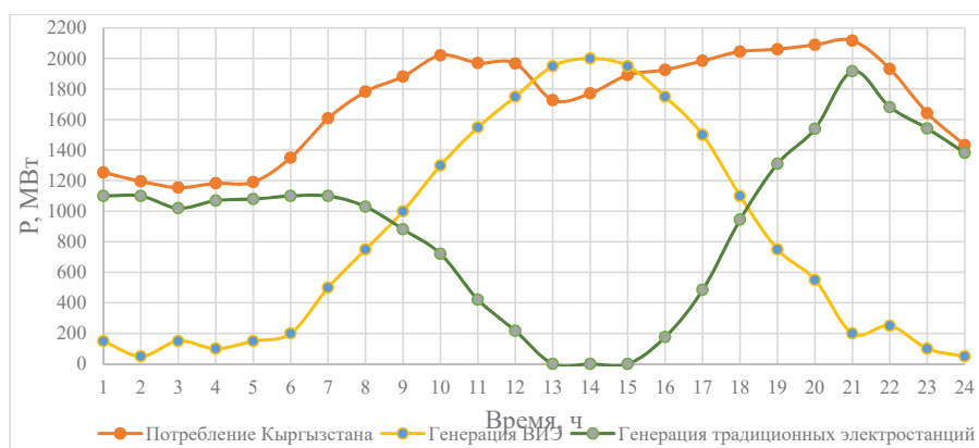
Рисунок 3 – Сценарий с максимальной генерацией ВИЭ 2 ГВт для летнего режима Кыргызстана
