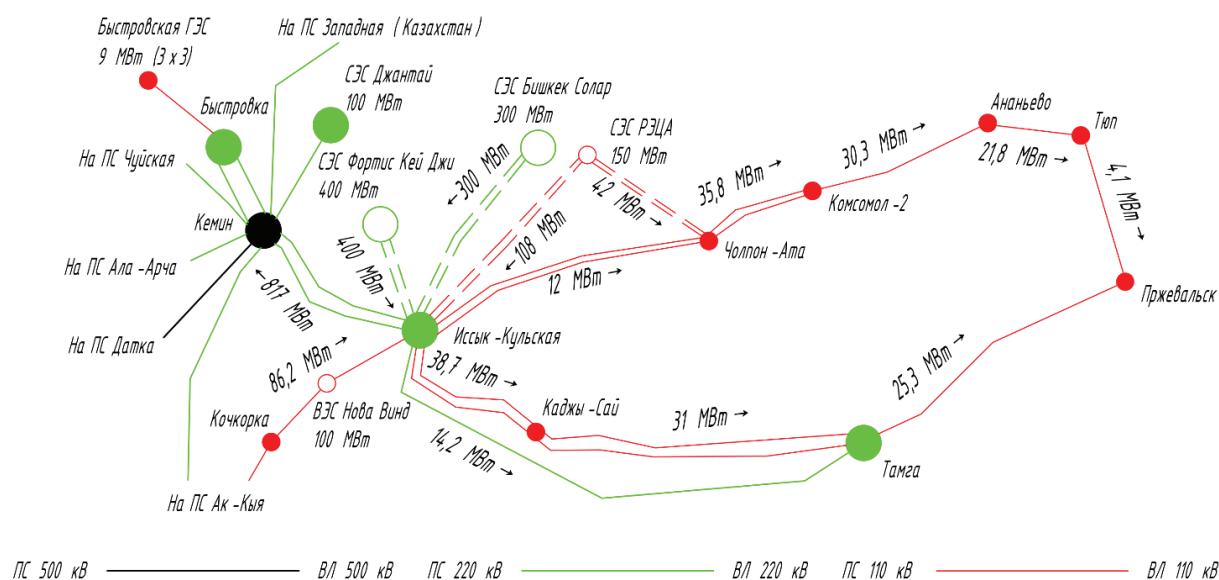
Рисунок 4 – Результаты расчета установившегося режима для летней максимальной генерации на объектах ВИЭ
